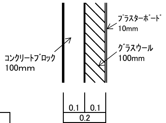
壁断面図
